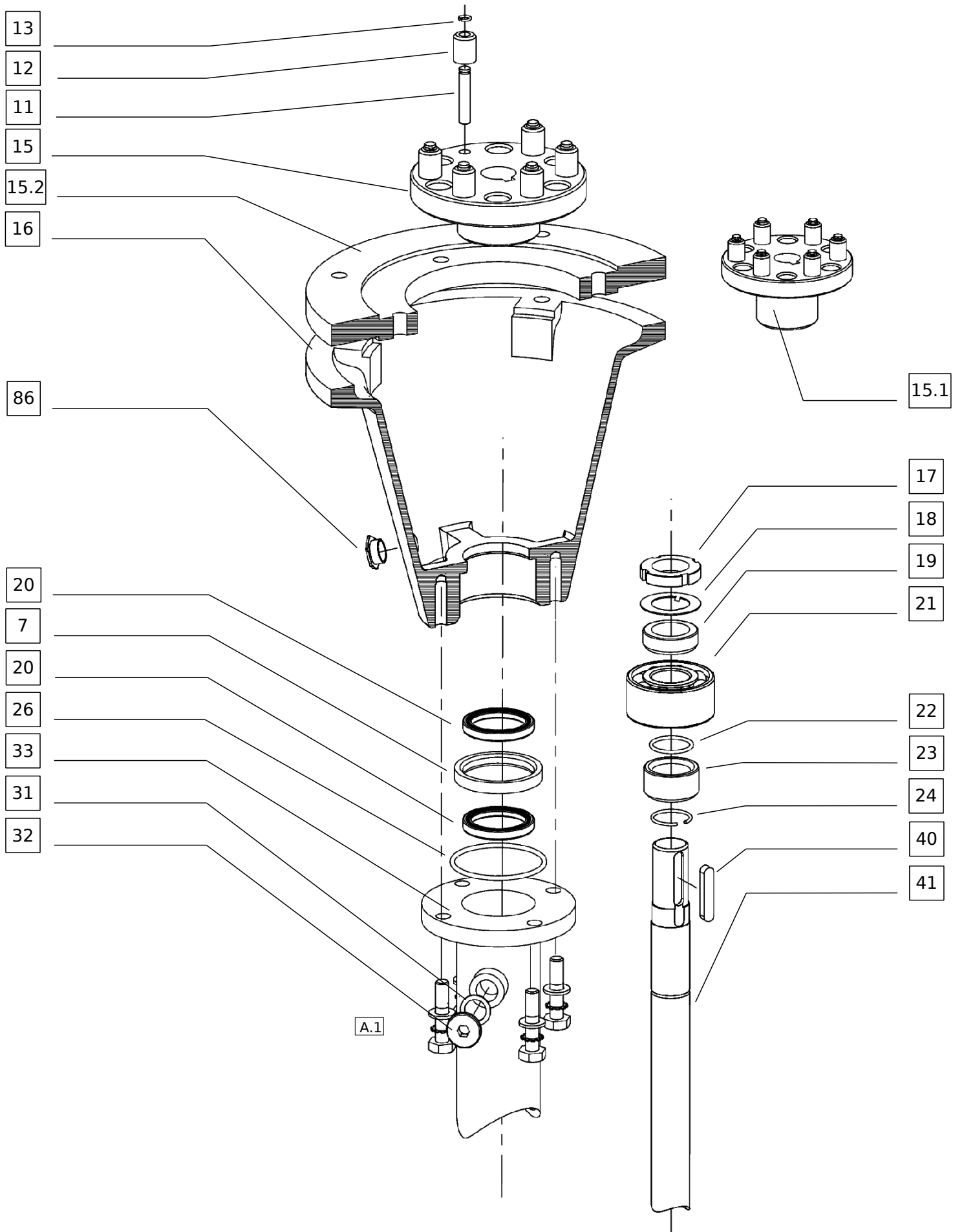
15.1 Kupplungshälfte Pumpe für 7.5kW Motor 15.2 Zwischenflansch für 7.5kW Motor
